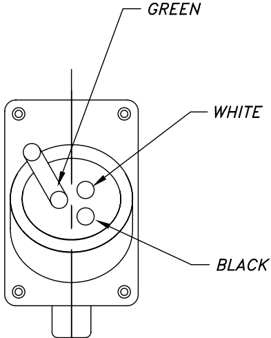
VIEW A-A BOX WIRING
