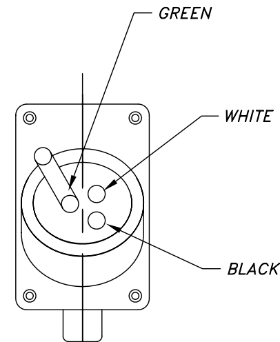
VIEW A-A BOX WIRING
